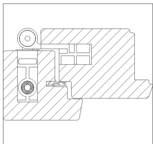
Applicazione singola guarnizione
