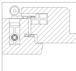
Applicazione doppia guarnizione
